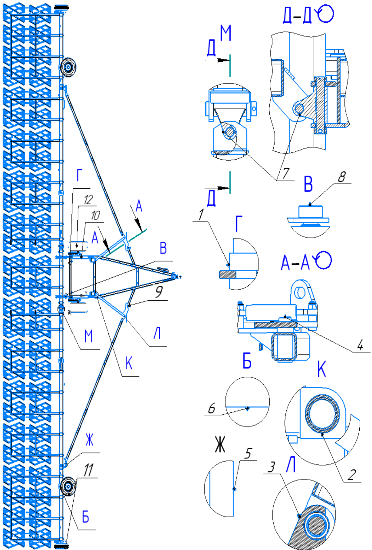
Рисунок 18 – Схема смазки
