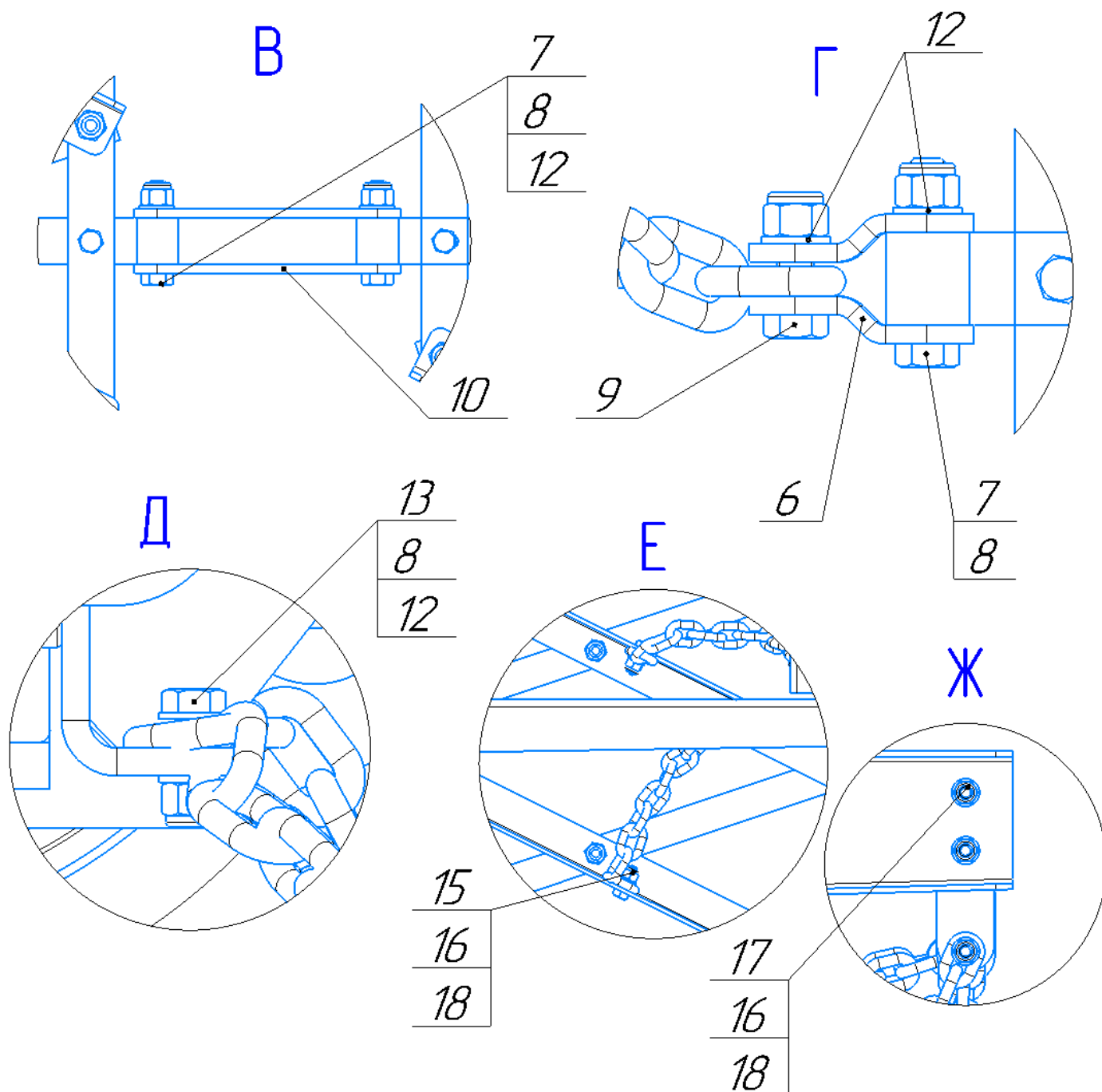
Рисунок 9 – Борона БЗС-1
