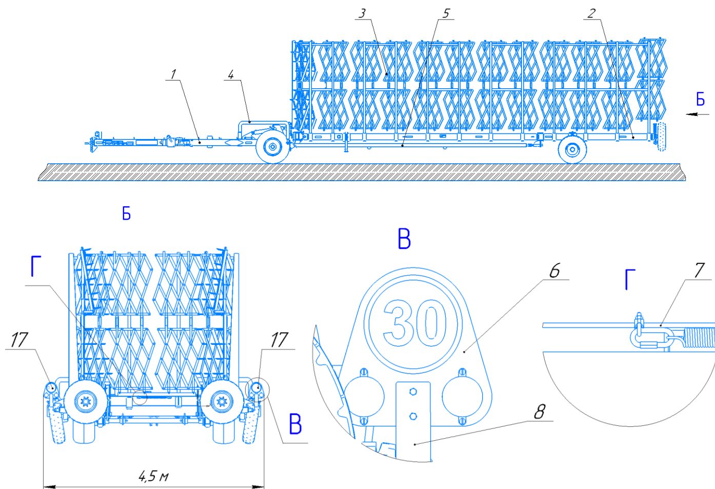
Рисунок 11 – Транспортное положение бороны
