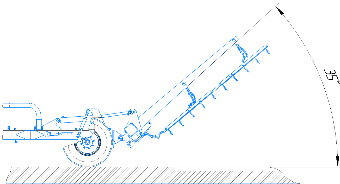
Рисунок 15 – Подъем борон для очистки зубьев
