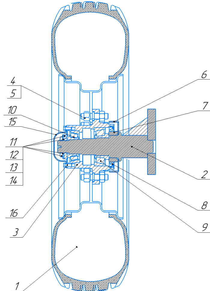
Рисунок 7 – Колесо ходовое
