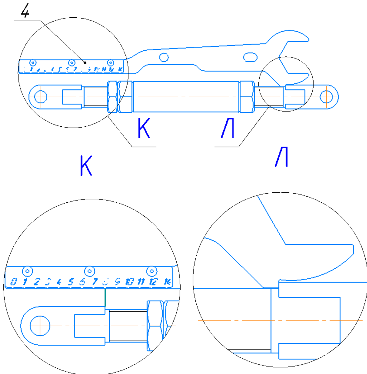
Рисунок 13 – Регулируемые опорные стойки
