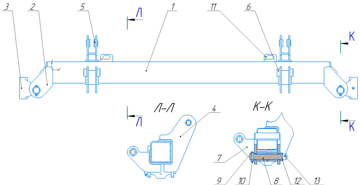
Рисунок 5 – Брус центральный
