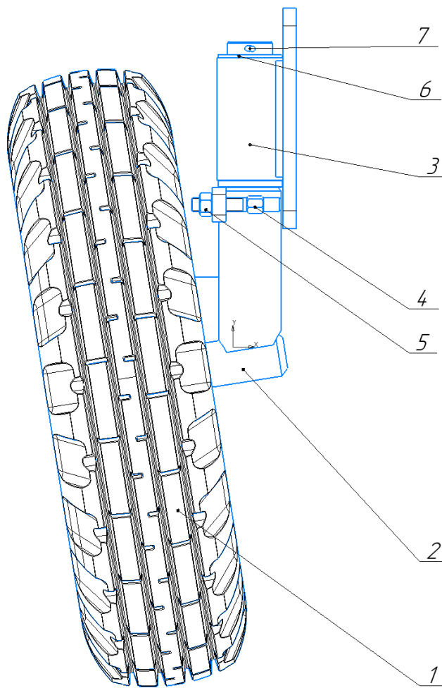
Рисунок 8 – Колесо транспортное
