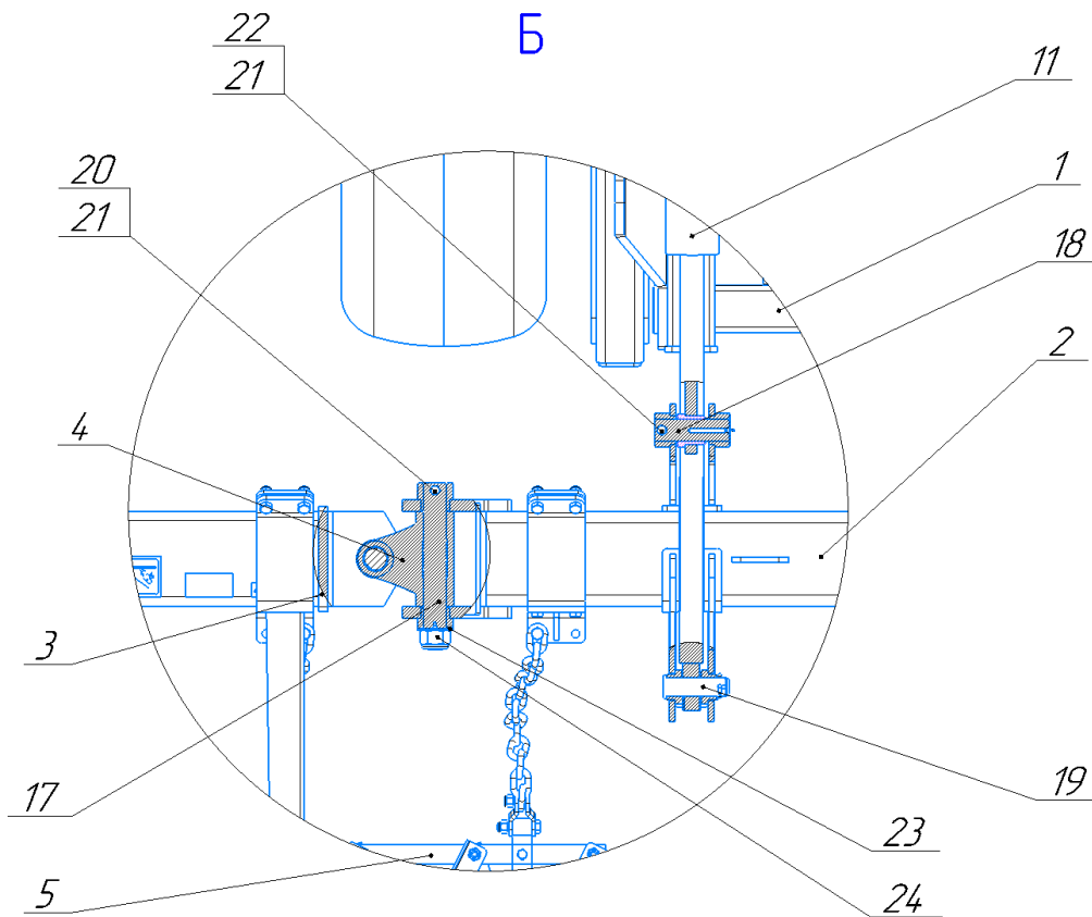
Рисунок 1 – Устройство бороны (рабочее положение)
