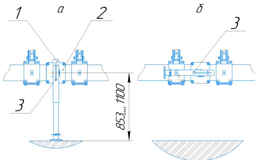
Рисунок 12 – Регулируемые опорные стойки
