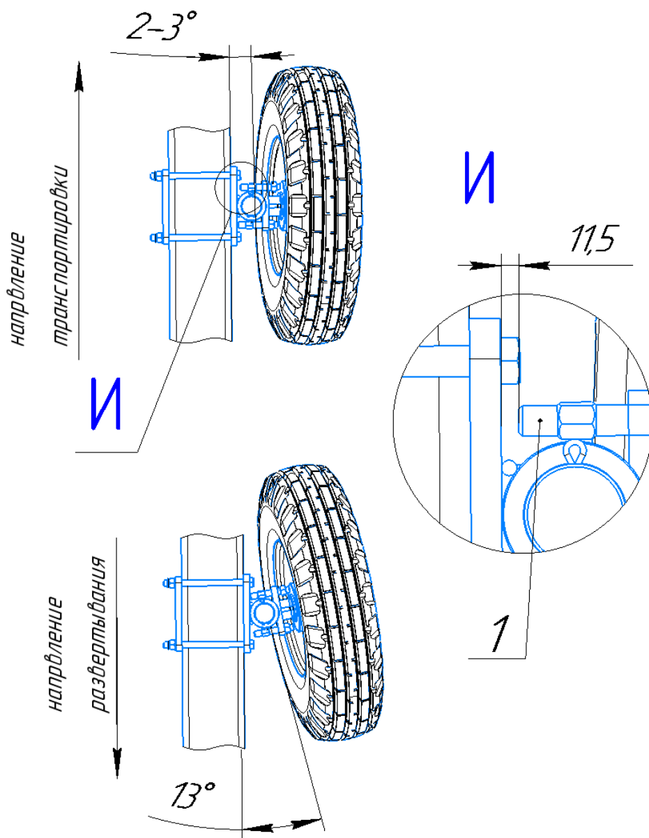
Рисунок 14 – Регулировка схождения транспортных колес 1 – болт регулировочный.
