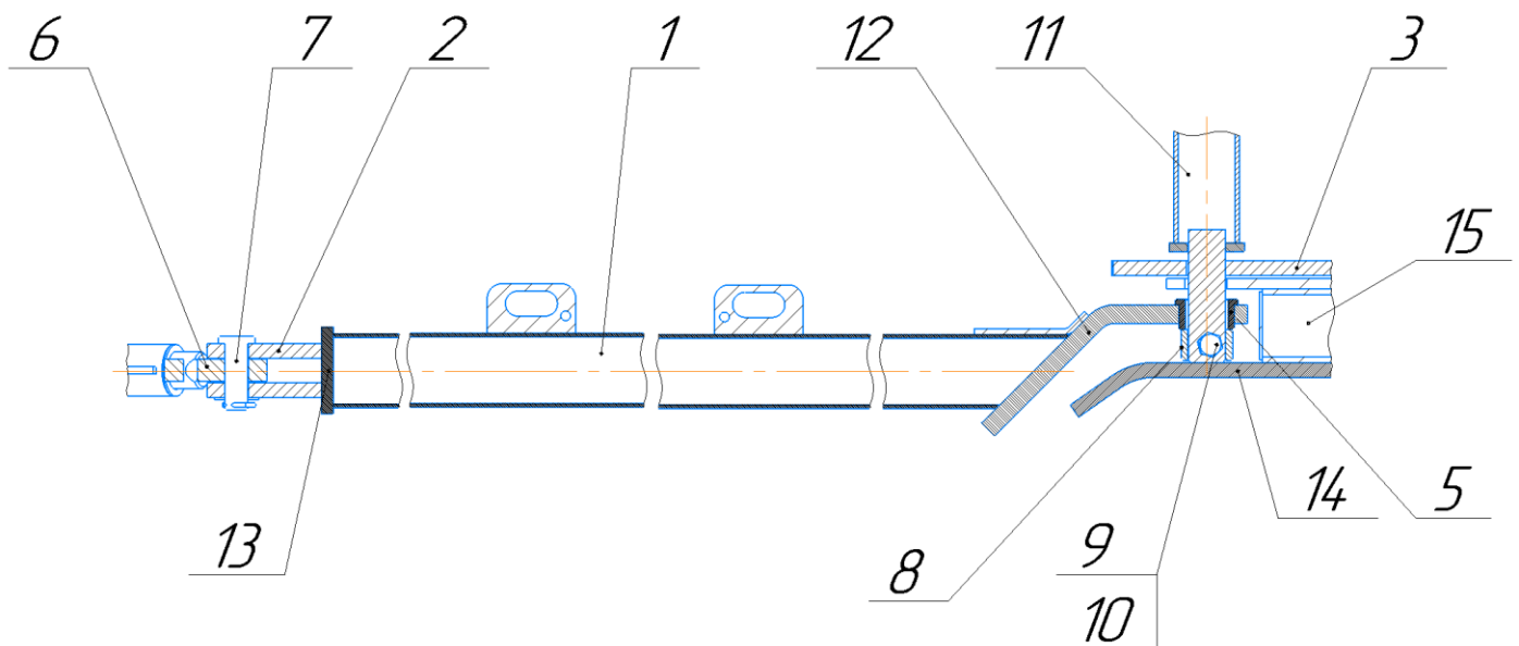
Рисунок 10 – Растяжка длинная
