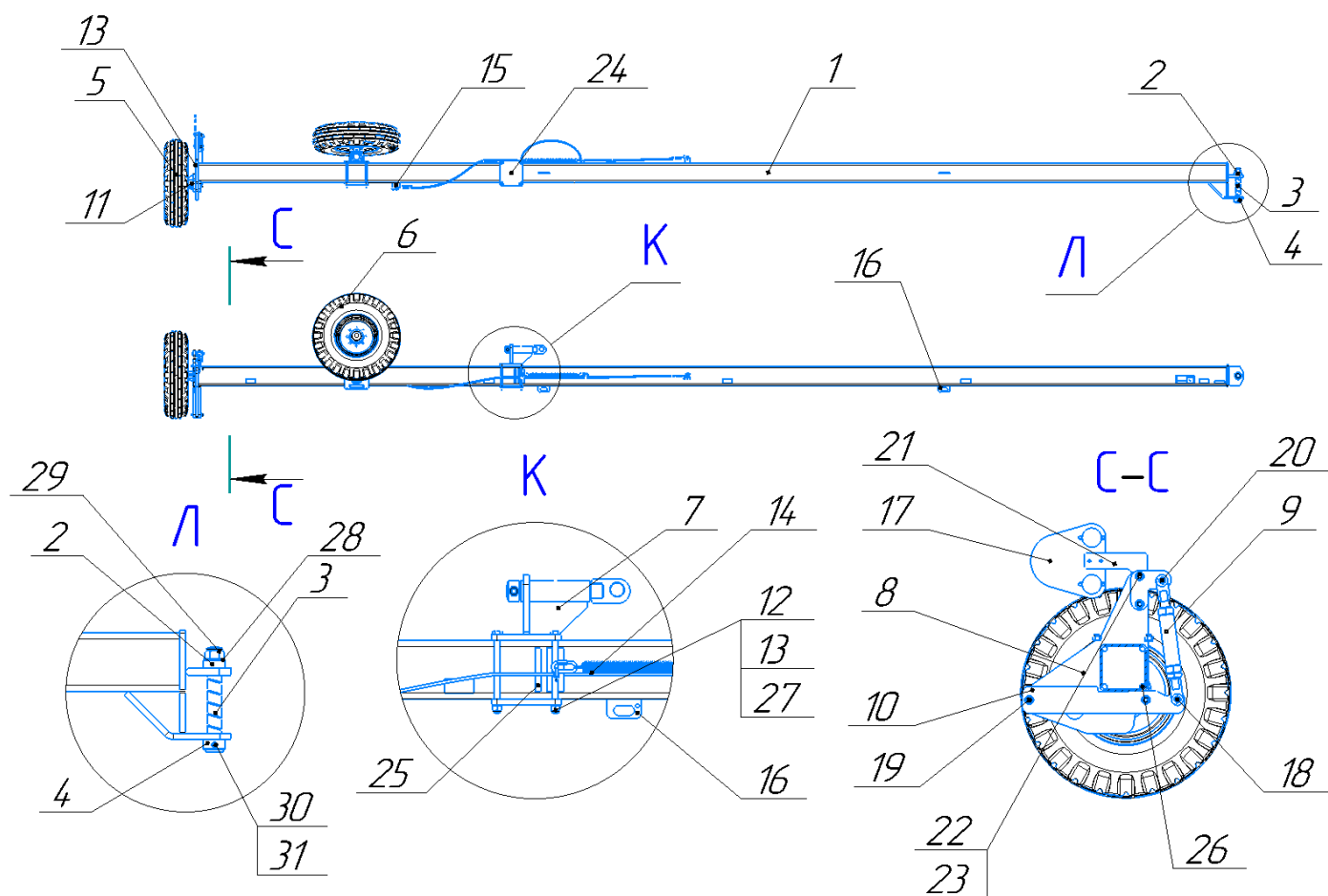
Рисунок 6 – Брус крайний
